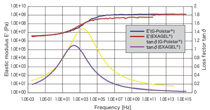
Mastercurve(23°C)
